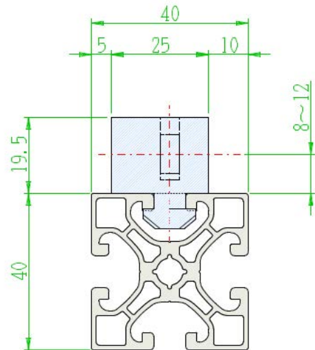
取付時寸法図
