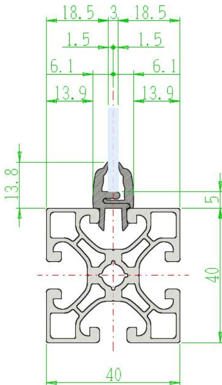
パネル厚3mmの場合
