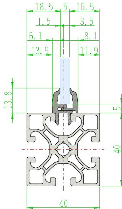
パネル厚5mmの場合
