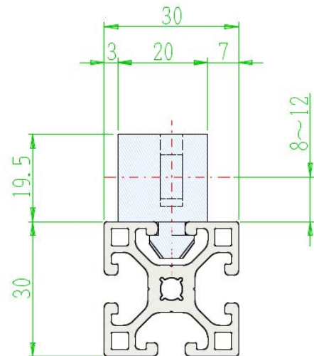
取付時寸法図
